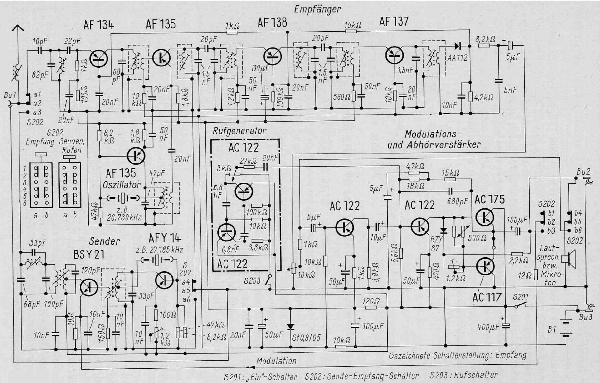
Bild 139. Schaltung des Handfunksprechgerätes für das 27-MHz-Band
