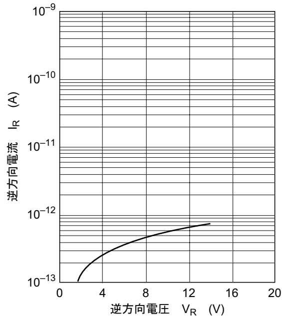
图1. 逆方向特性
